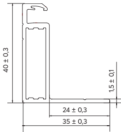
Rahmenprofil
